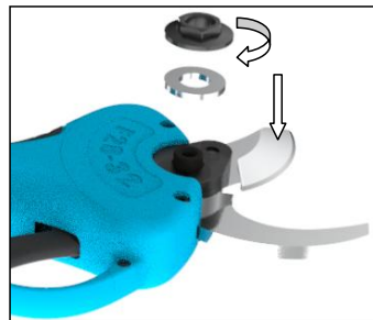
10.按照图示放入平面滚针轴承,并拧上锁紧螺母。
