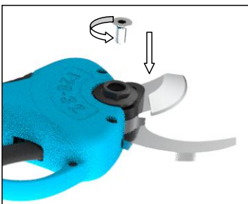
11.按照图示逆时针方向拧上M5内六角沉头螺丝。
