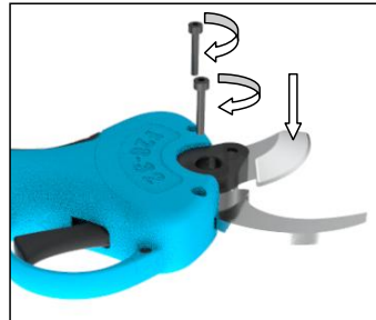
8.按照图示拧上M3内六角螺丝。
